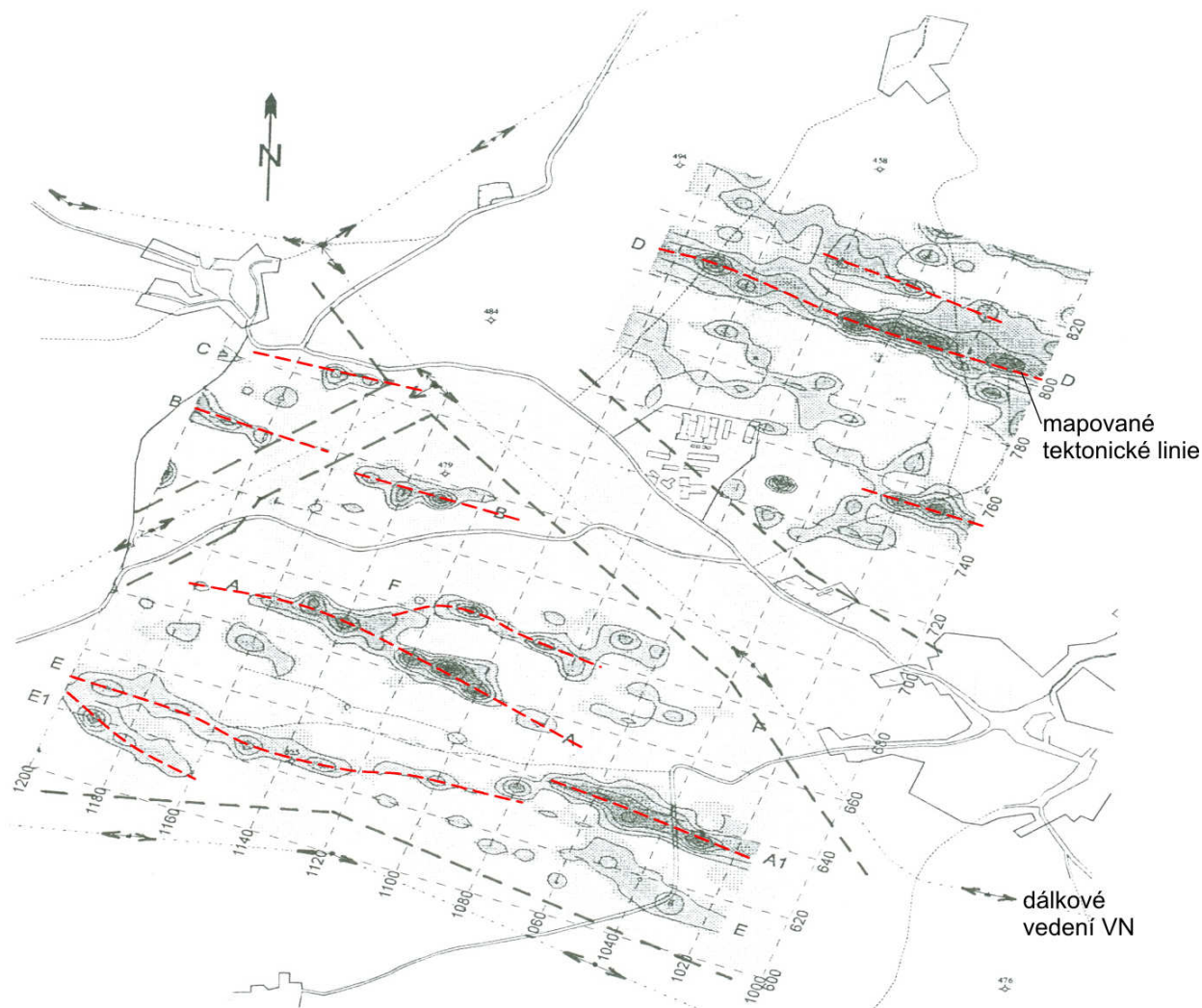
Obr. 3.5. Mapa vodivostních indicií tektonických poruch z metody velmi dlouhých vln
