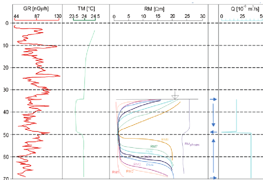
Obr. 3.5. Stratifikace dvou systémů oběhu podzemních vod, vzestupné i sestupné proudění podle karotáže
