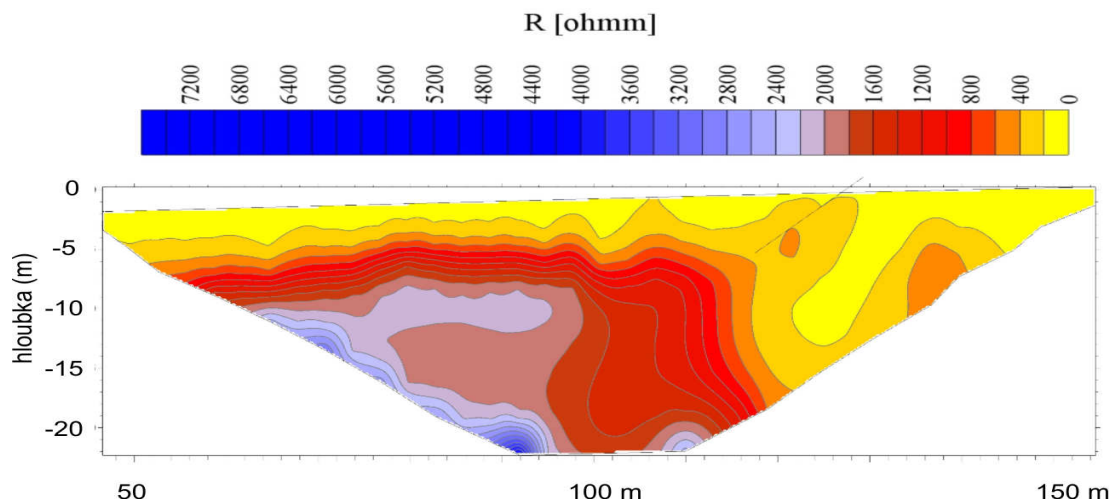
Obr. 3.2. Odporový řez stanovený multielektrodotým uspořádáním při průzkumu mocnosti propustných fluvialních sedimentů
