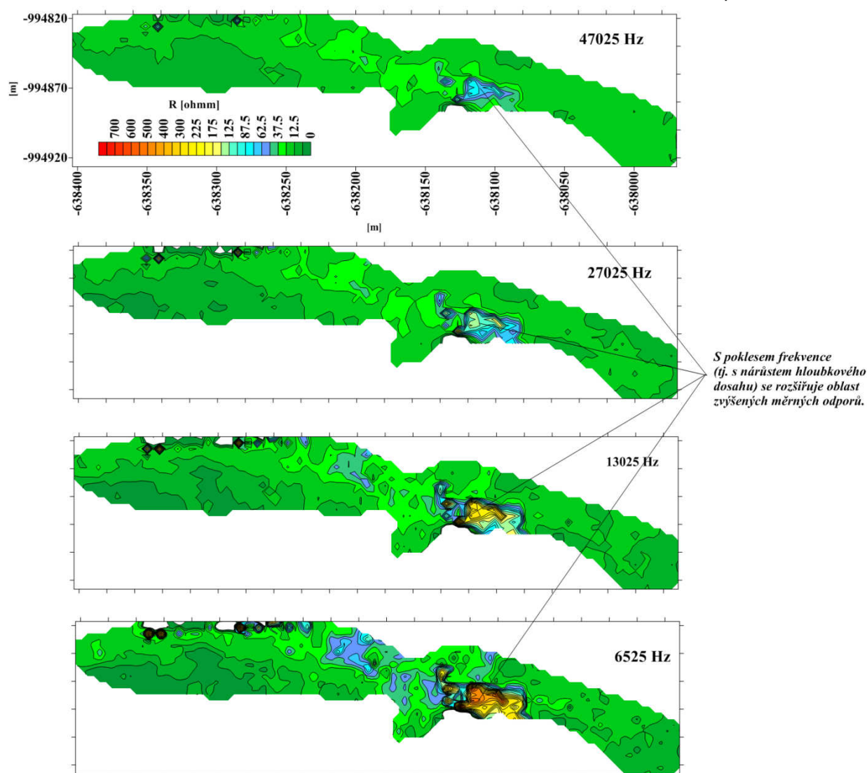
Obr. 2.7. Mapy izoliní měrných odporů DEMP pro 4 různé frekvence zdrojového EM pole
