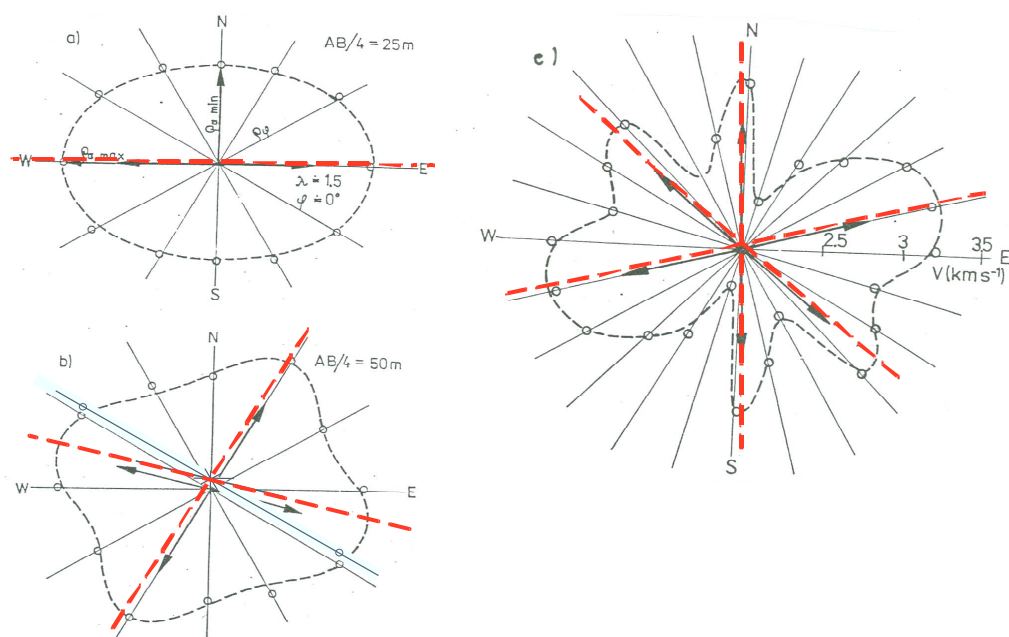
Obr. 3.8. Zjištění směru puklinatosti odporovým (a, b) a seismickým (c) radiálním měřením (směr tektoniky je zakreslen červenými přerušovanými čarami: a) prostředí s jedním převládajícím směrem poruch, b) se dvěma, c) se třemi směry)
