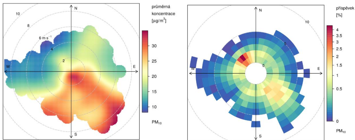
Obr. 59: Koncentrační růžice (vlevo) a vážená koncentrační růžice (vpravo) pro PM 10 , stanice BBNV, aglomerace Brno CZ06A, 2011-2016
