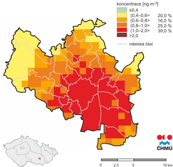
Obr.26: Pětiletý průměr ročních průměrných koncentrací benzo[a]pyrenu, aglomerace Brno CZ06A, 2007–2011
