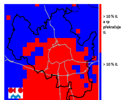
Obr. 43: Příspěvek českých zdrojů (silniční doprava a lokální vytápění) k ročnímu průměru benzo[a]pyrenu, aglomerace Brno CZ06A
