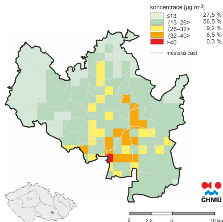
Obr.31: Pětiletý průměr ročních průměrných koncentrací \text{NO}_2 , aglomerace Brno CZ06A, 2012–2016
