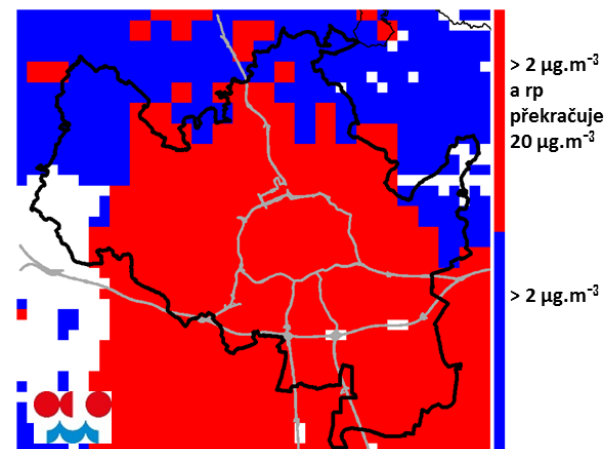
PM 2,5 - oblasti s příspěvkem > 2 µg.m -3 primární PM 2,5 z REZZO 3 - lokální vytápění
