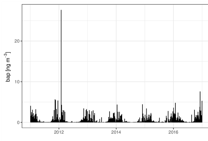
Obr. 57: Časová řada denních B[a]p, stanice BBNA, aglomerace Brno CZ06A, 2011–2016
