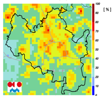
Obr. 43: Příspěvek českých zdrojů (silniční doprava a lokální vytápění) k ročnímu průměru benzo[a]pyrenu, aglomerace Brno CZ06A
