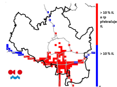
B[a]P - oblasti s příspěvkem > 10 % IL REZZO 4 - silniční doprava
