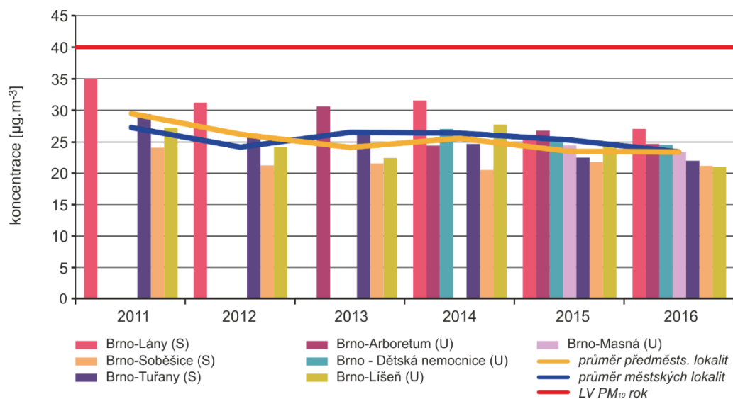
Obr. 8 : Průměrné roční koncentrace \text{PM}_{10} na městských a předměstských lokalitách, aglomerace Brno CZ06A, 2011–2016
