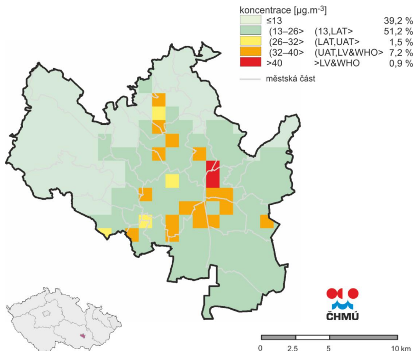
Obr. 29: Pole průměrné roční koncentrace \text{NO}_2 , aglomerace Brno CZ06A, 2016
