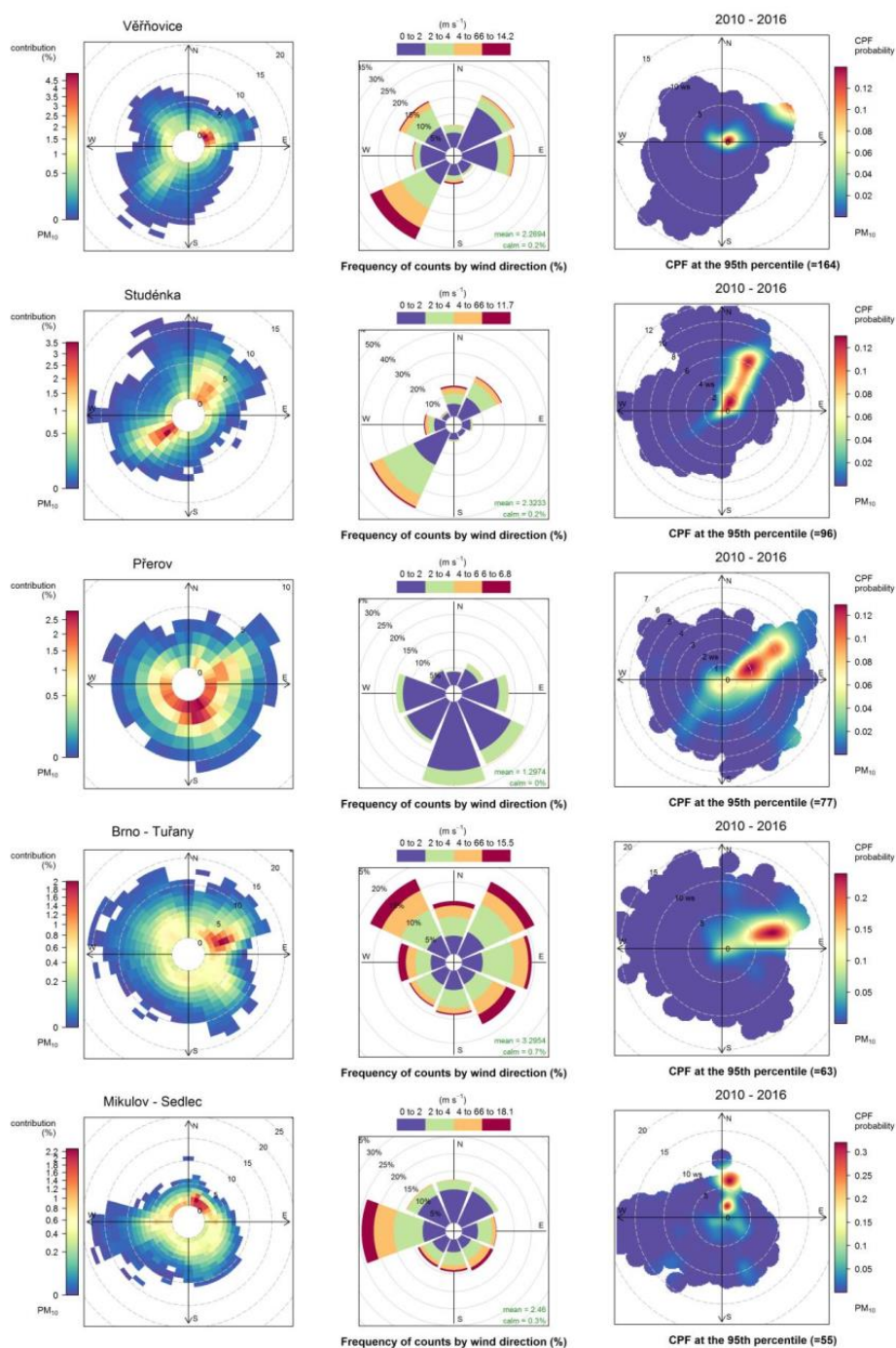
Obr. 33: Vážené koncentrační růžice (vlevo), větrné růžice (uprostřed) a pravděpodobnostní koncentrační růžice zobrazující směry větru s 5 % nejvyšších koncentrací PM_{10} (vpravo) v lokalitách Věřňovice, Studénka, Přerov, Brno-Tuřany a Mikulov-Sedlec, 2010–2016, převzato ze Skeřil (2017) 6
