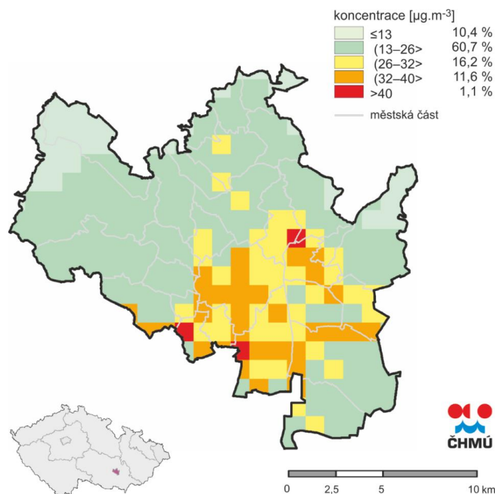
Obr. 30: Pětiletý průměr ročních průměrných koncentrací \text{NO}_2 , aglomerace Brno CZ06A, 2007–2011
