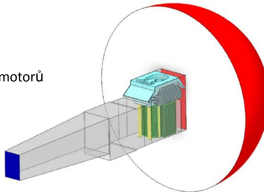
Obr. 14 Vzduchový chladicí systém motoru (modře – vstup vzduchu, červeně – výstup)
