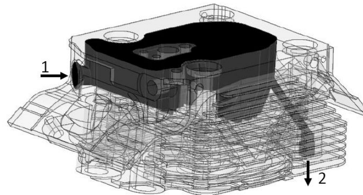
Obr. 11 Hlava motoru s olejovou lázní (1 – vstup oleje do lázně, 2 – výstup oleje z lázně)
