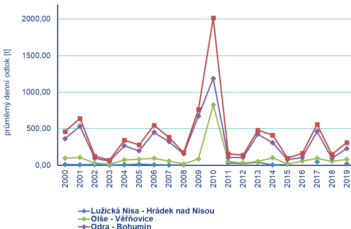
Obr. 8.8.2 Průběh ročních hodnot průměrného denního odtoku plavenin ve stanicích Odra – Bohumín, Olše – Věřňovice a Lužická Nisa – Hrádek nad Nisou.
