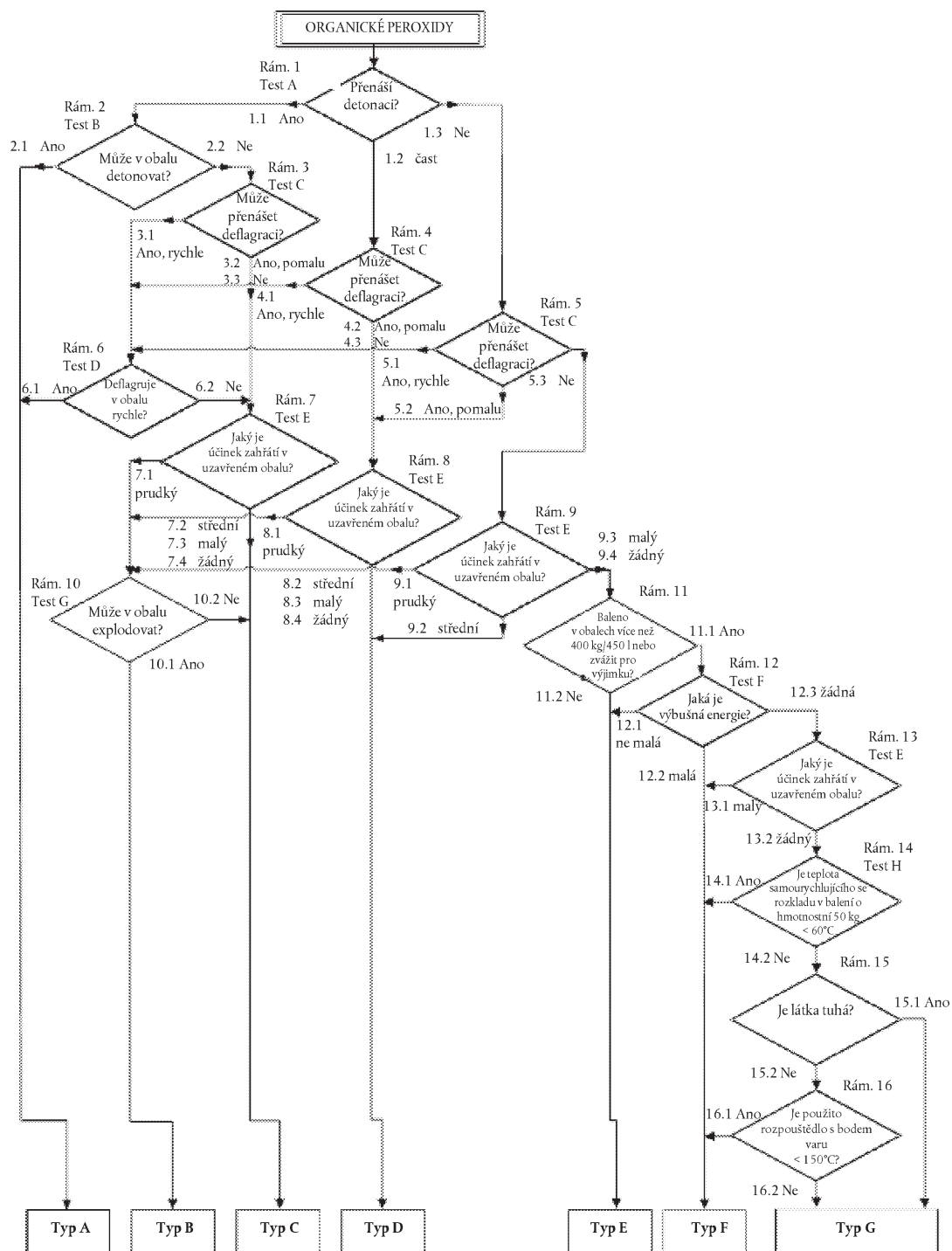
Obrázek 2.15.1 Organické peroxidy
